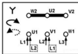
Sternschaltung
