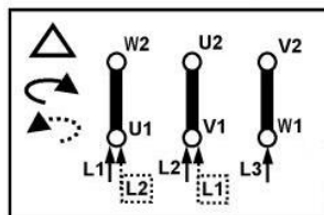
Dreieckschaltung
